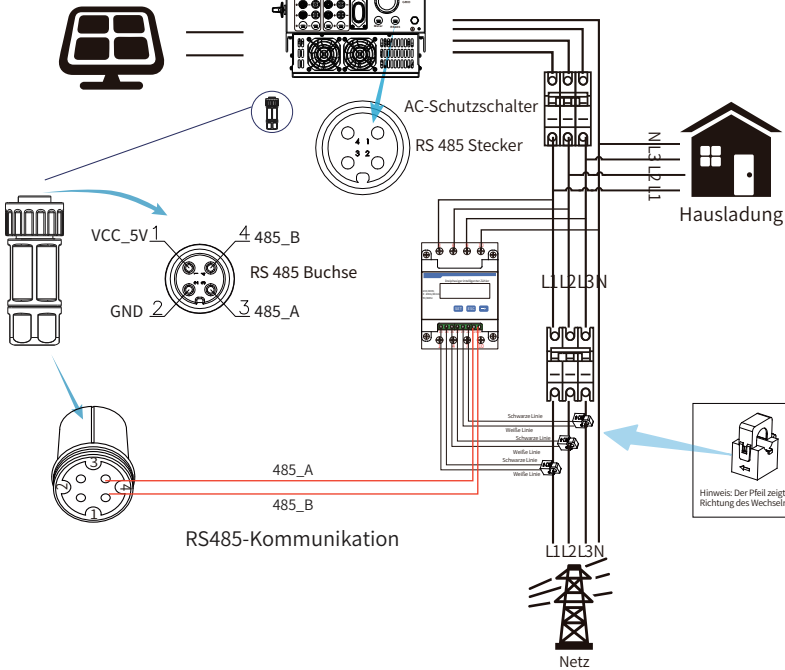
Abb. 7.14 Anschlussplan des CHINT-Zählers
